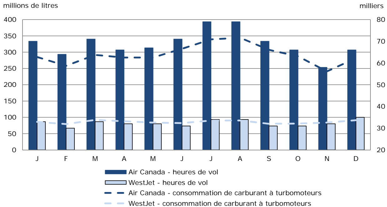
Graphique 6 Heures de vol et consommation de carburant à turbomoteurs, Air Canada et WestJet, janvier à décembre 2011
